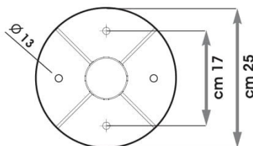
Base fissaggio - Base plate
