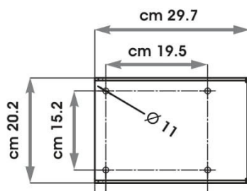
Base fissaggio - Base plate
